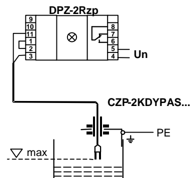
Przykład sygnalizacji poziomu max
