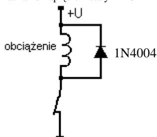
Rysunek 2 – zabezpieczenie przy zasilaniu napięciem stałym DC
