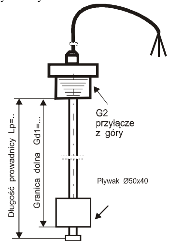
Rysunek ofertowy czujnika jedno lub wielo-punktowego CPPG-...-...
