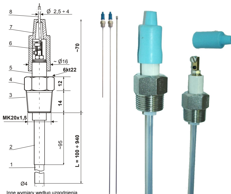
Inne wymiary według uzgodnienia Wymiary i widok czujnika poziomu cieczy i ciał sypkich - odmiana CZP-1-MK20x1,5
